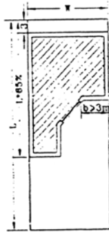
دیگرام حداقل فاصله دیوار دارای پنجره از بر قطعه
