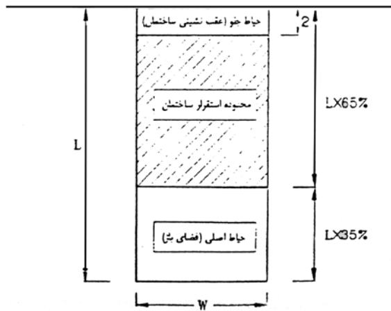
محدوده استقرار و حناکر مجاز بیشروی ساختمان در طول زمین در قطعات جنوبی
