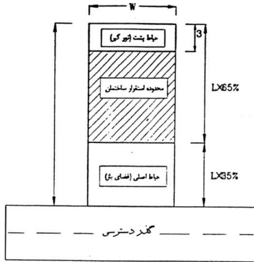
محدوده استقرار و حناکر مجاز بیشروی ساختمان در طول زمین در قطعات شمالی
